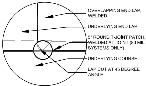
TJ-2: END LAP BOTTOM T-JOINT
