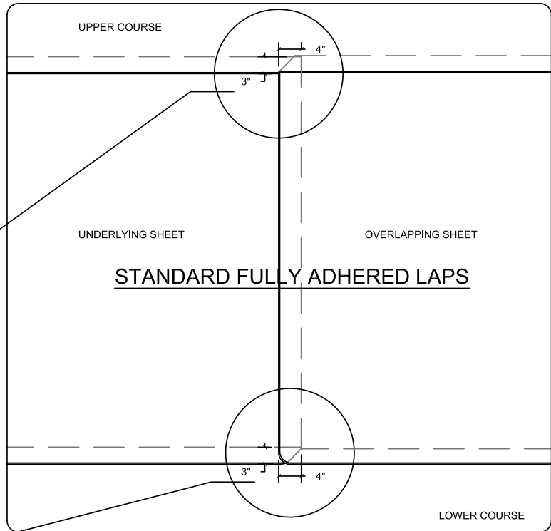
TJ-1: END LAP TOP T-JOINT
