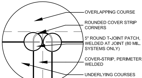
CS-1: COVER-STRIP TOP T-JOINT
