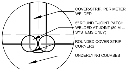
CS-2: COVER-STRIP BOTTOM T-JOINT
