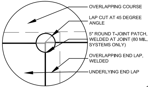
TJ-1: END LAP TOP T-JOINT
